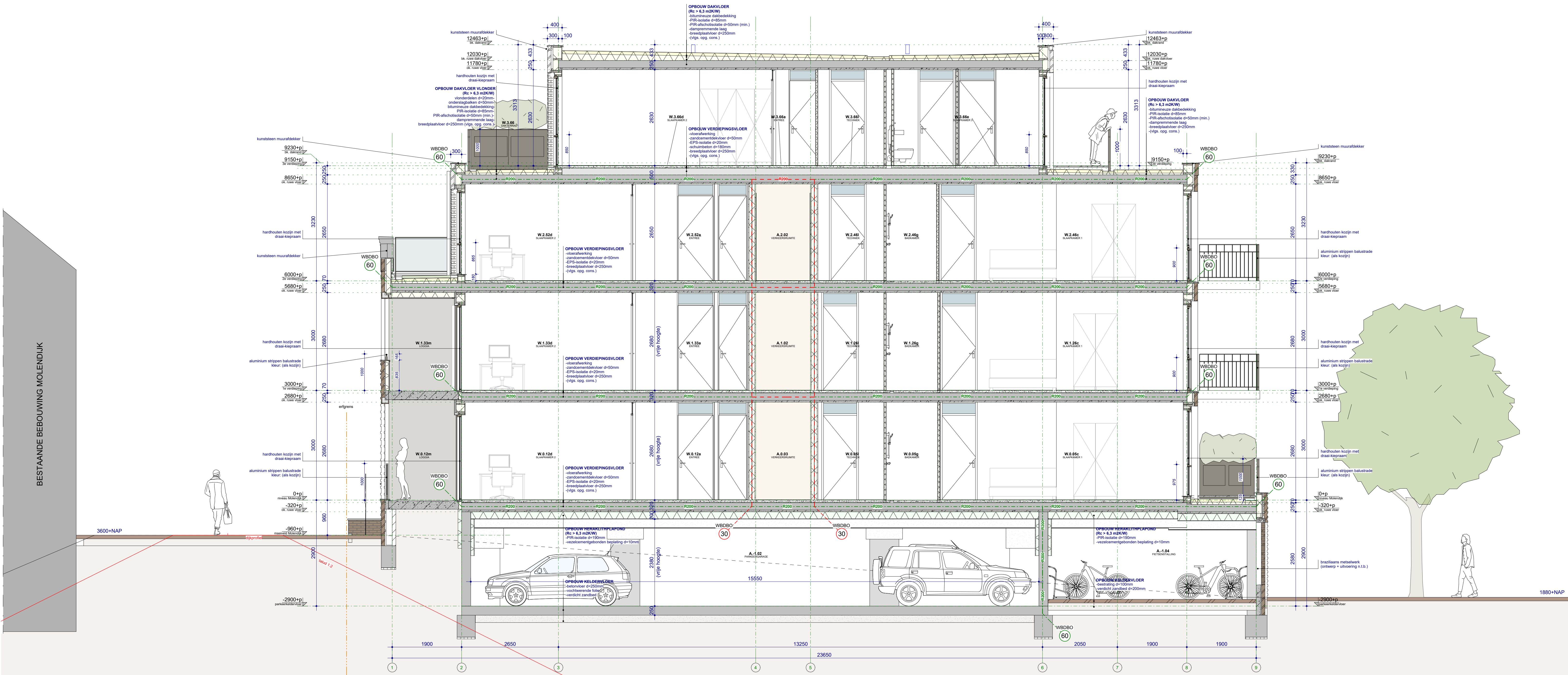
DOORSNEDE A-A
