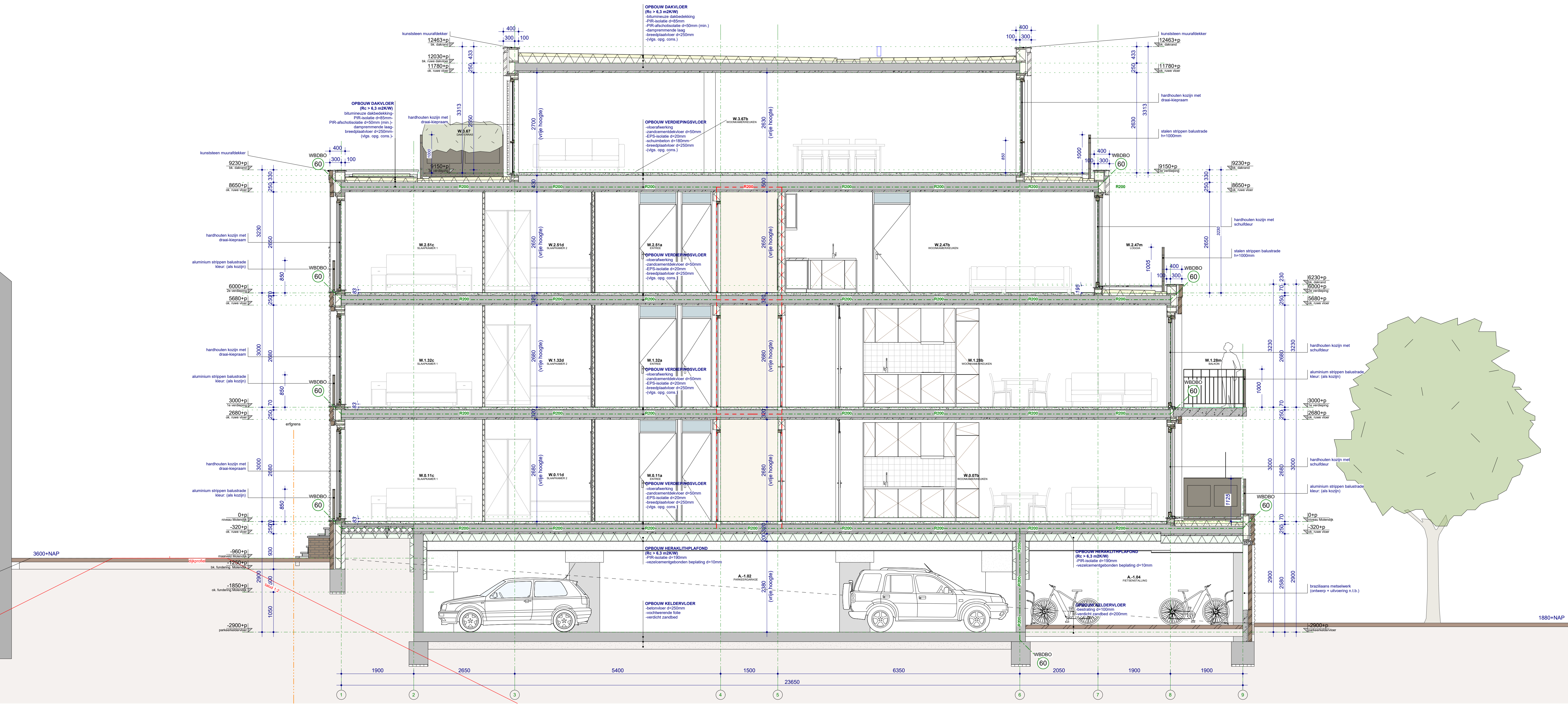
DOORSNEDE B-B
