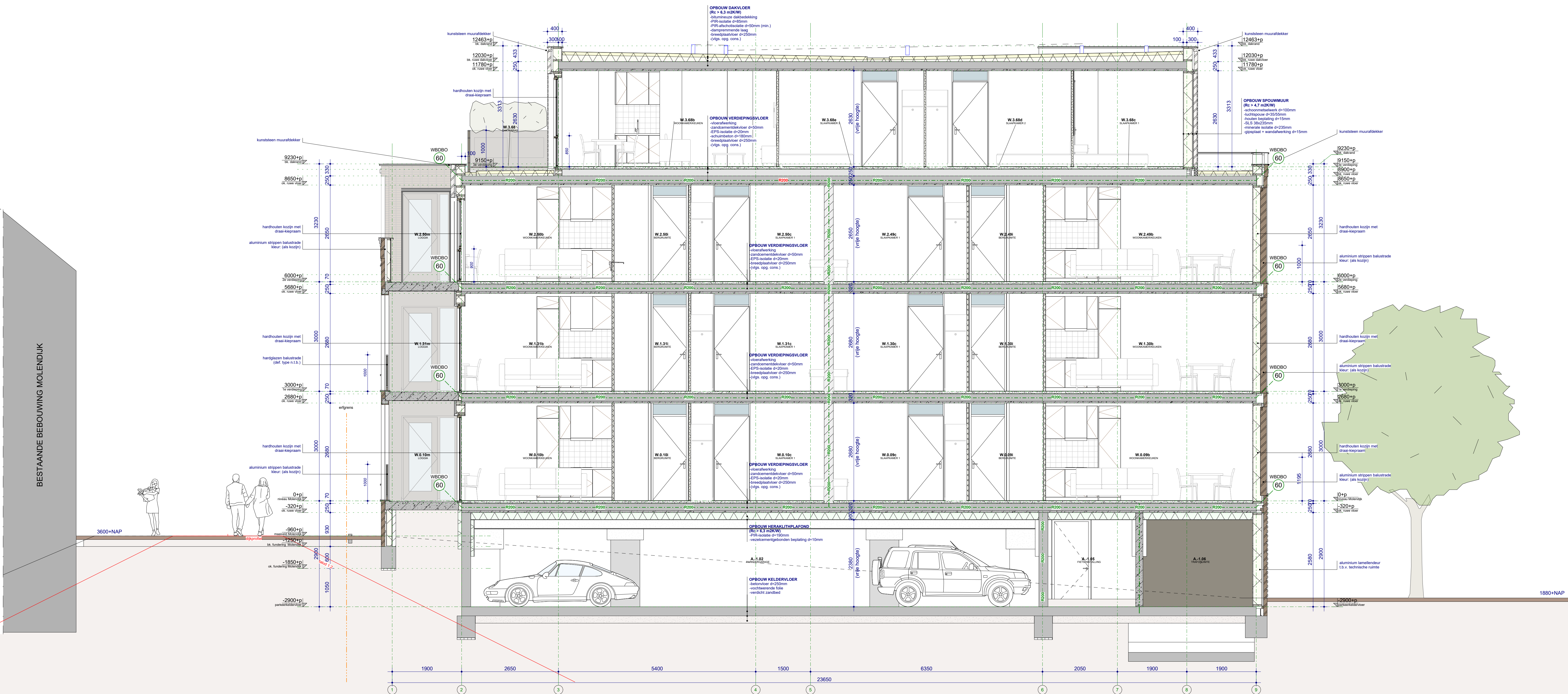
DOORSNEDE C-C
