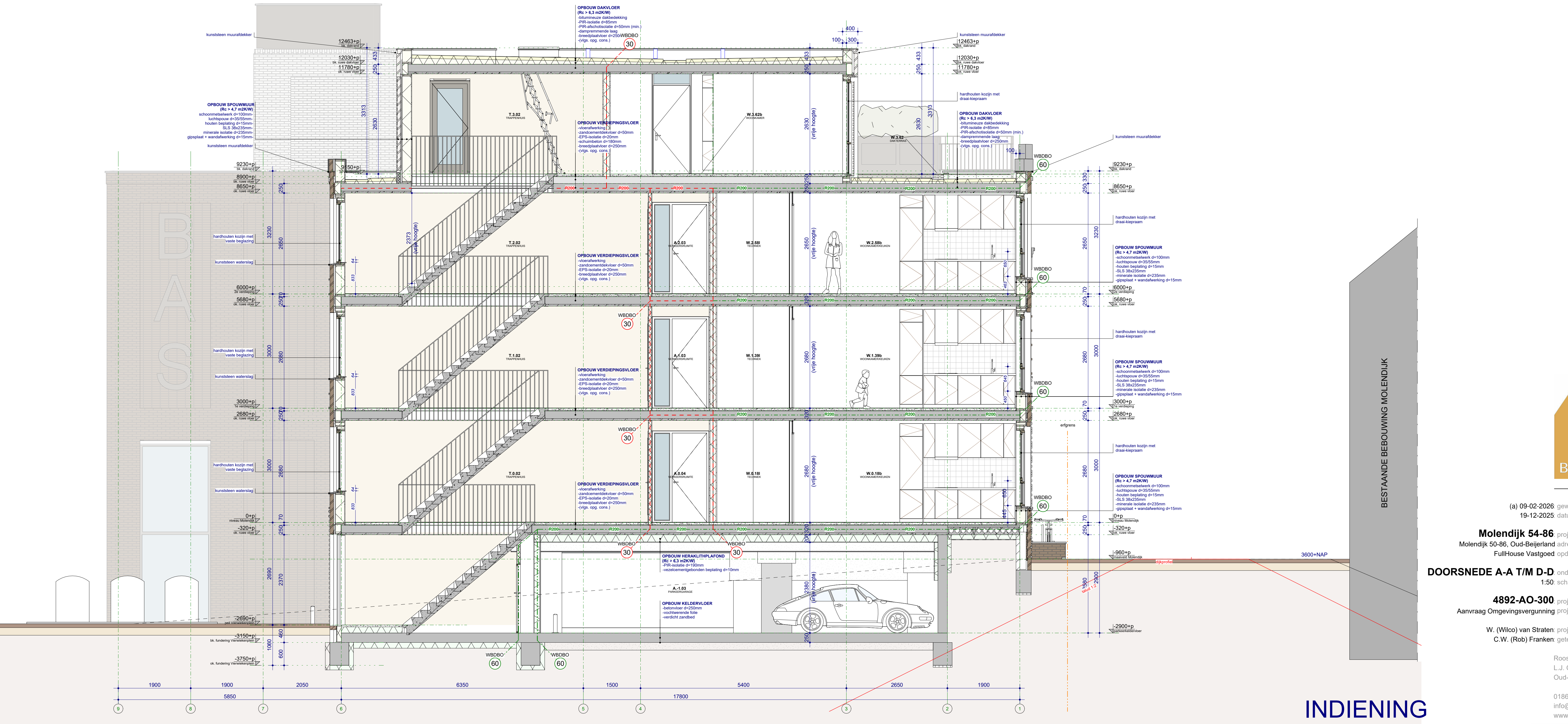
DOORSNED D-D
