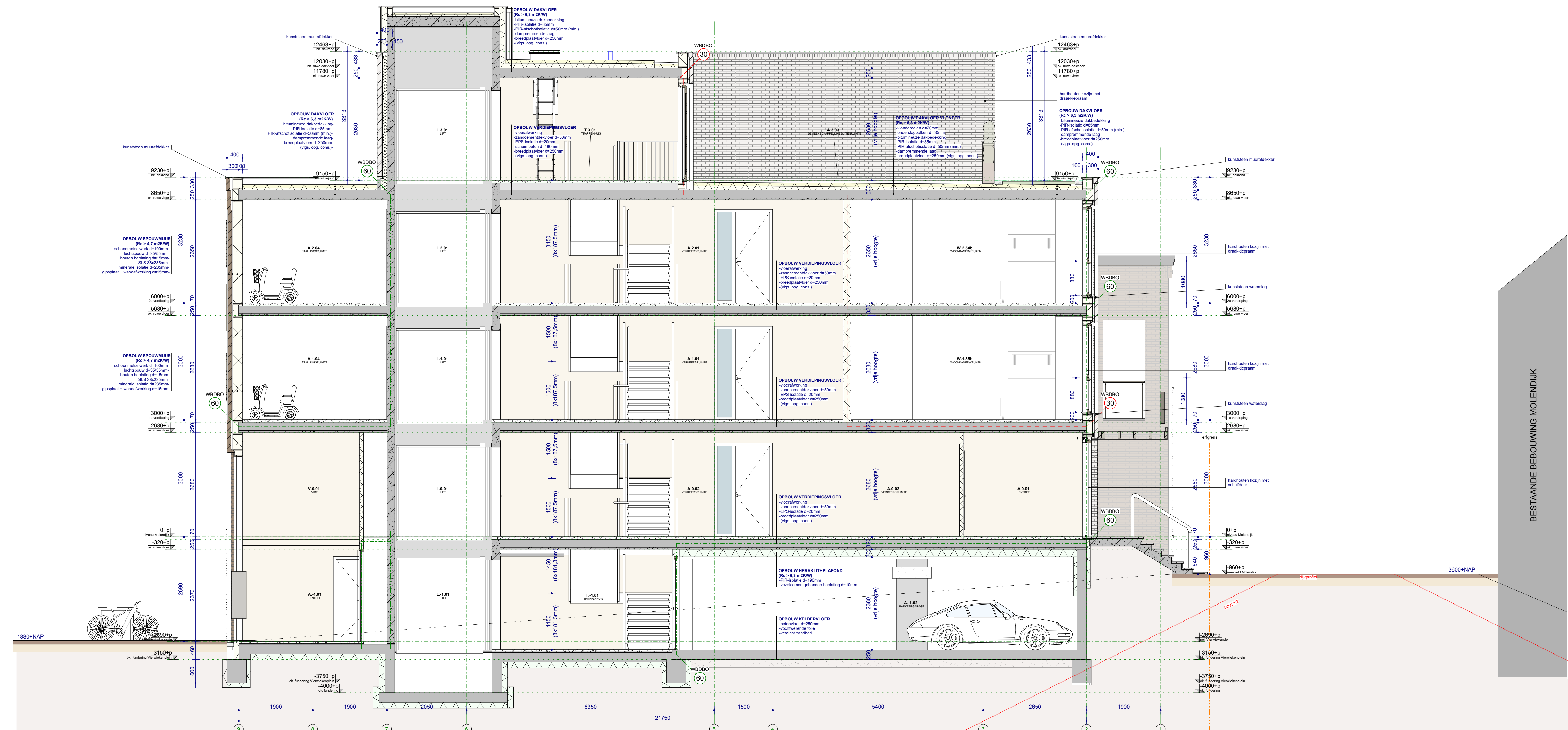
DOORSNEDE G-G
