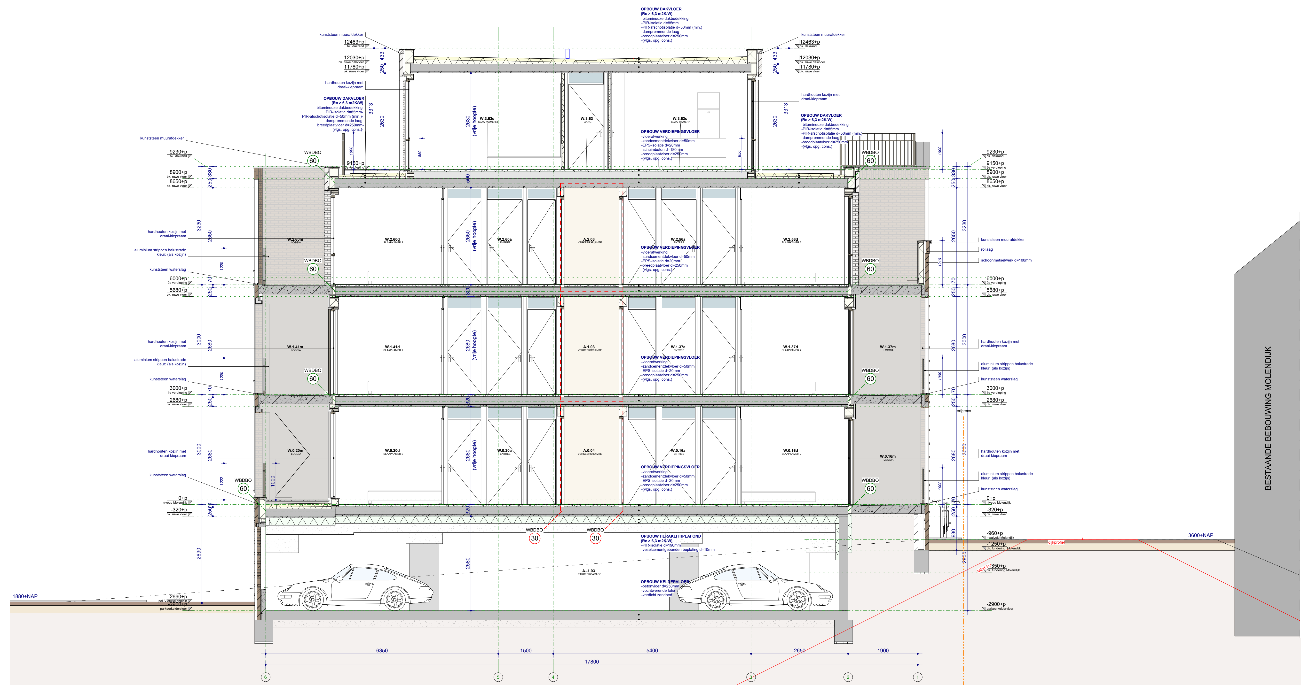
DOORSNEDE F-F
