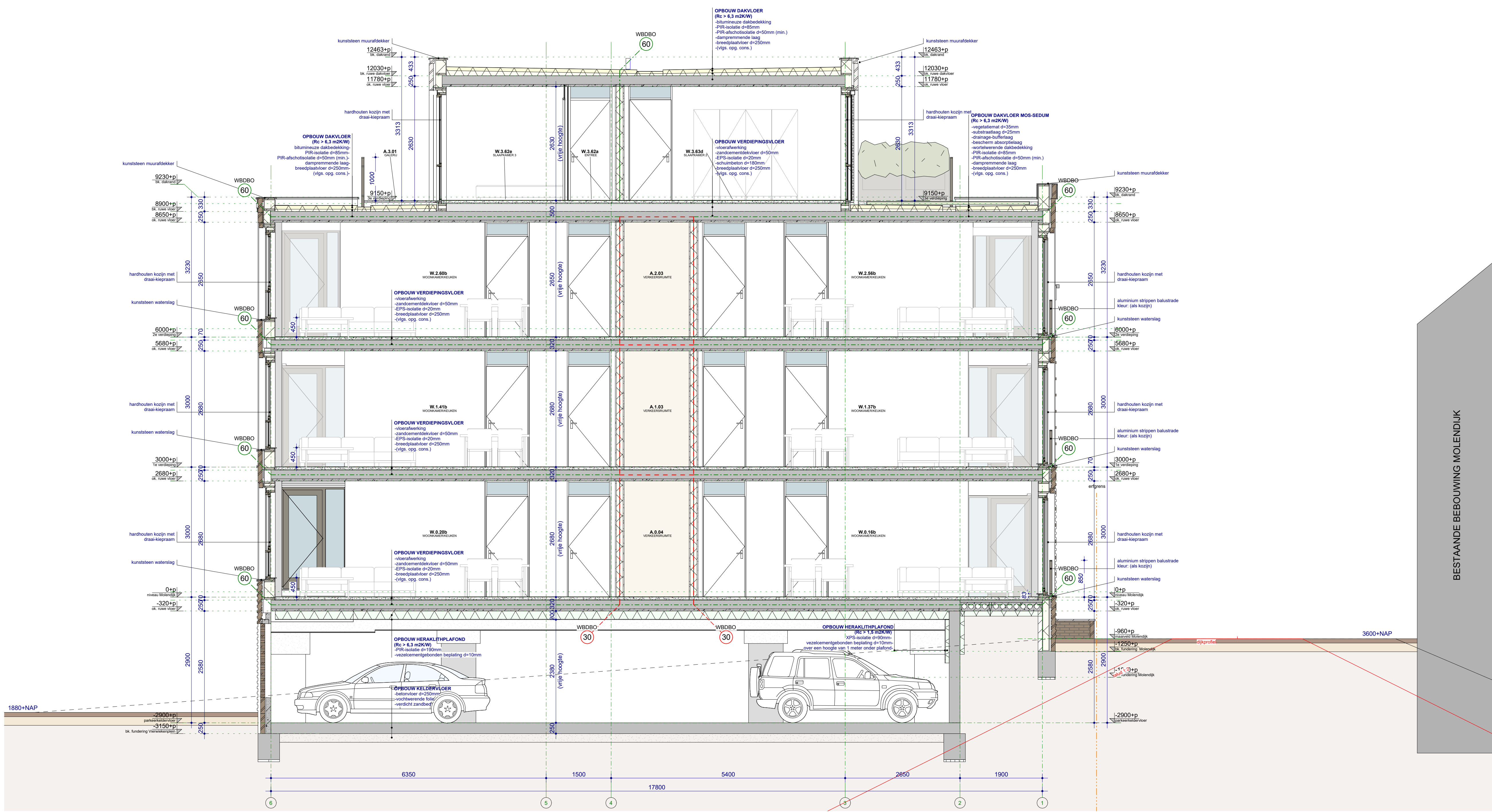
DOORSNEDE E-E
