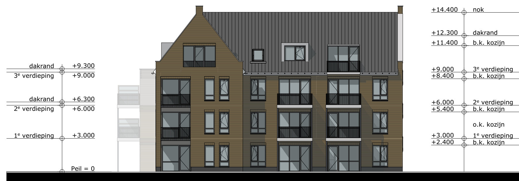
NOORDGEVEL
