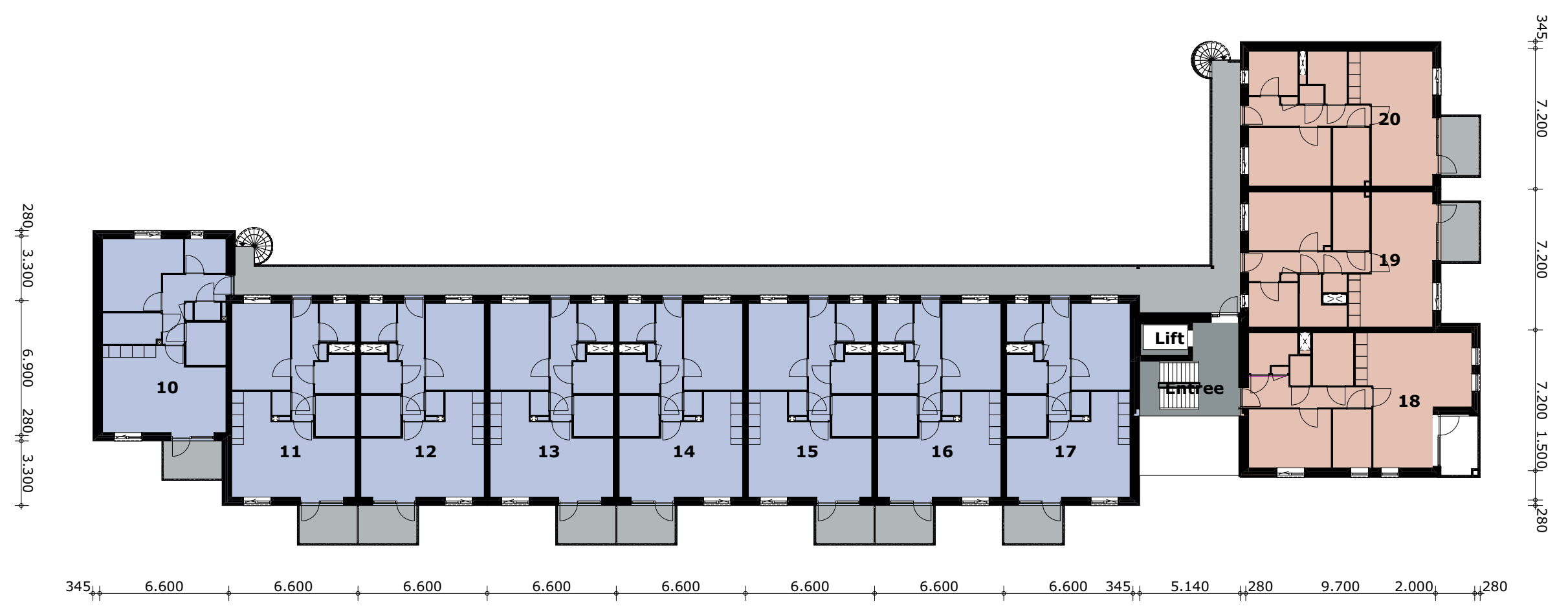
1E VERDIEPING
