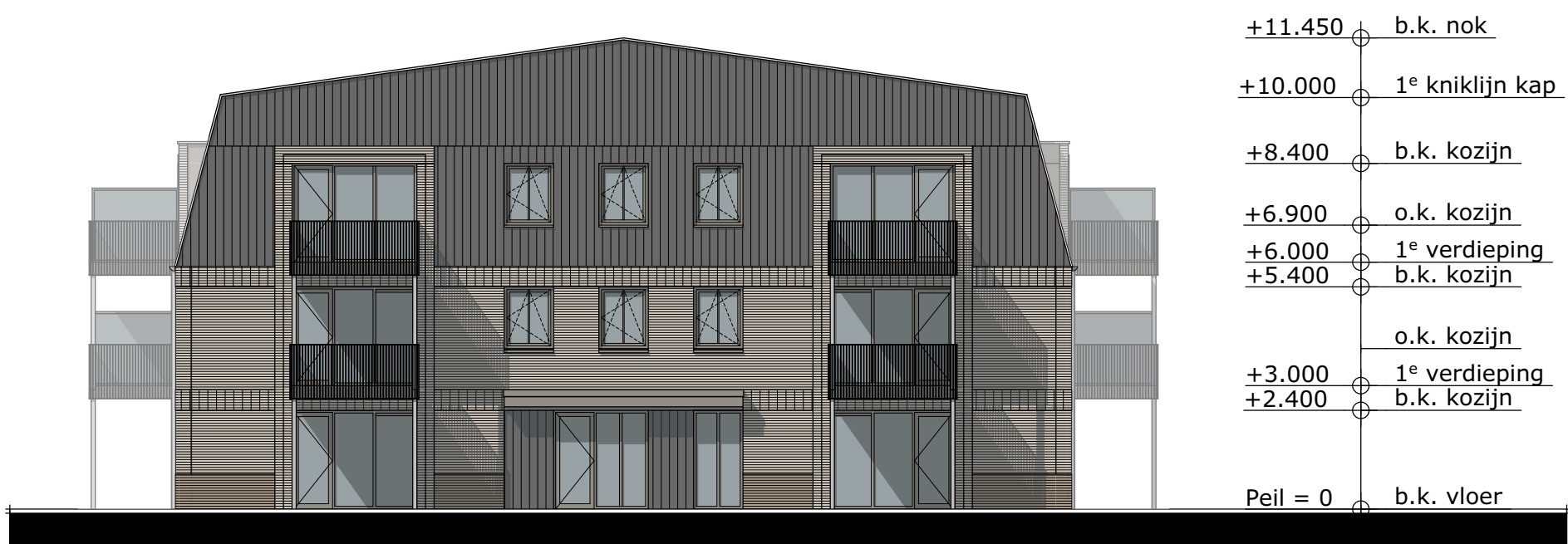
NOORD-WESTGEVEL
