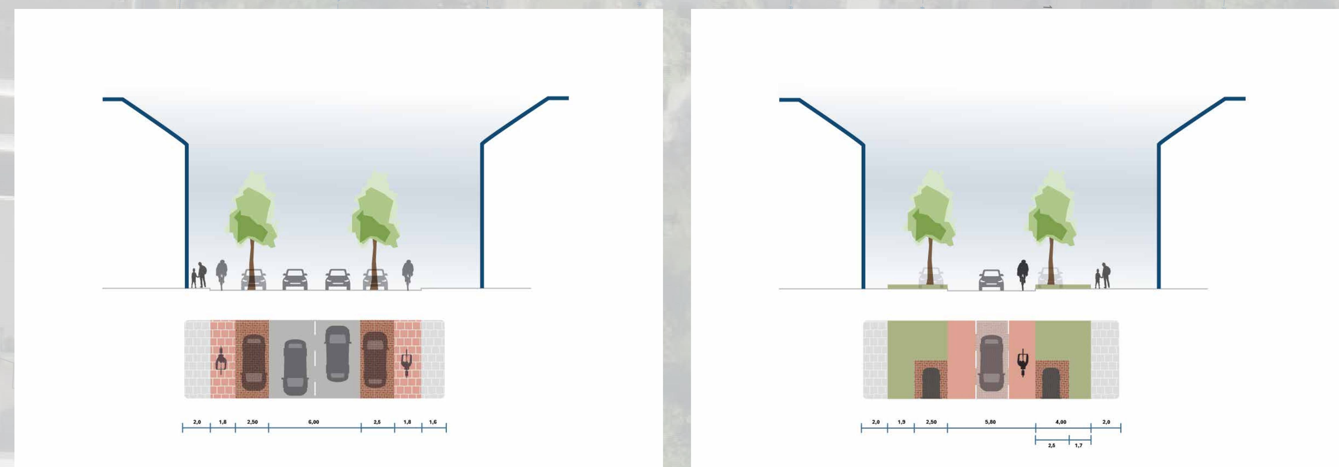
Dwarsprofiel Burg. de Zeeuwstraat huidige situatie - beoogde situatie
