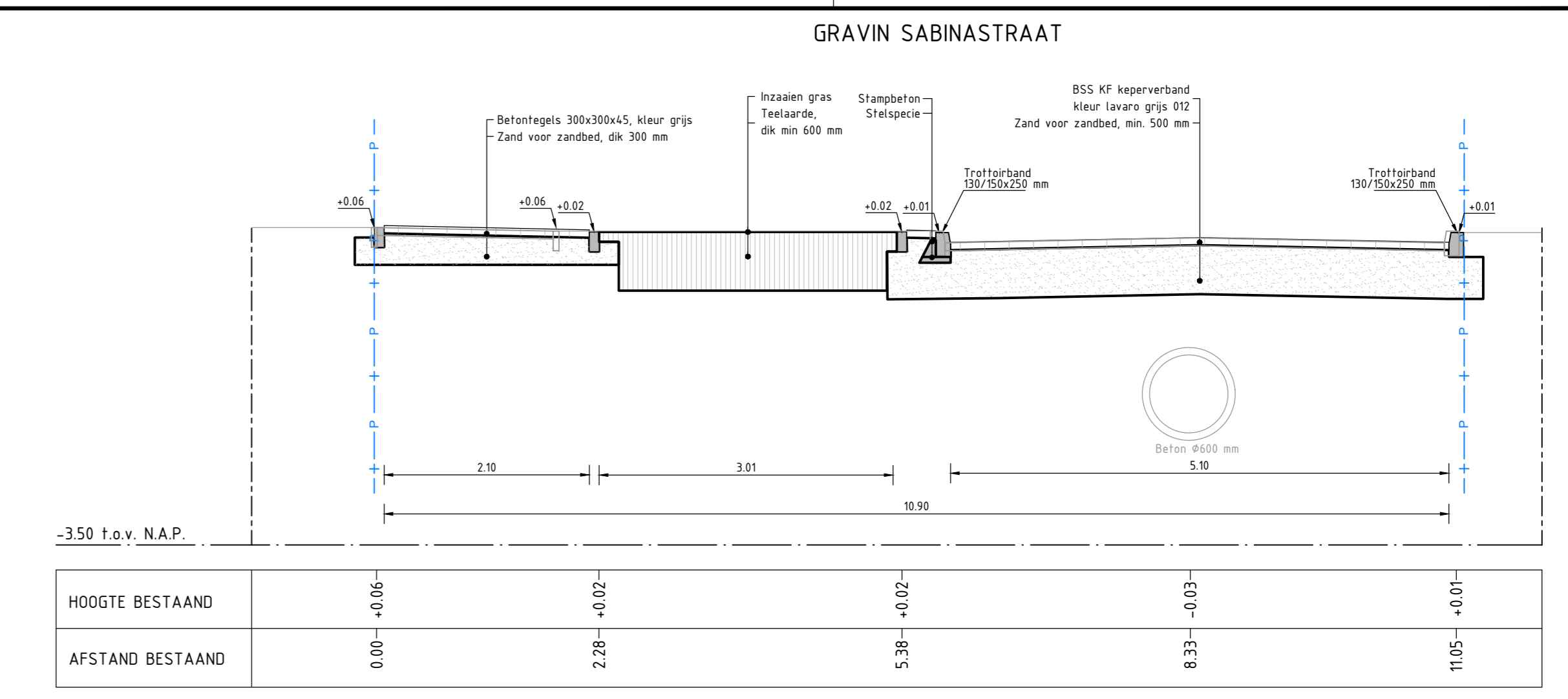
DOORSNEDE 8-8 SCHAAL 1:50
